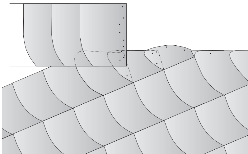
Zakončení u hřebene s přesahem.
