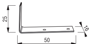
Příchytka hřebenáče
