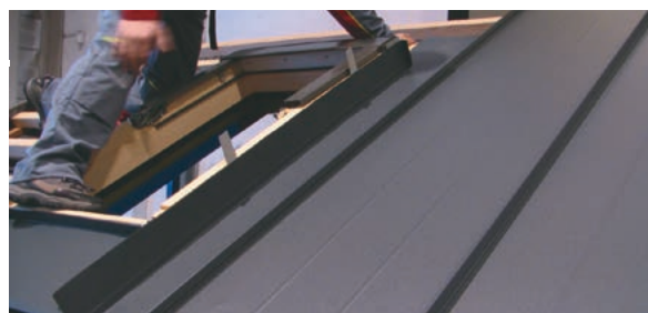
Zhotovení čelového oplechování z hladkého plechu a jeho přichycení k větracím profilům a oknu. Osazení druhé boční šablony, vytvarované do potřebného tvaru.
