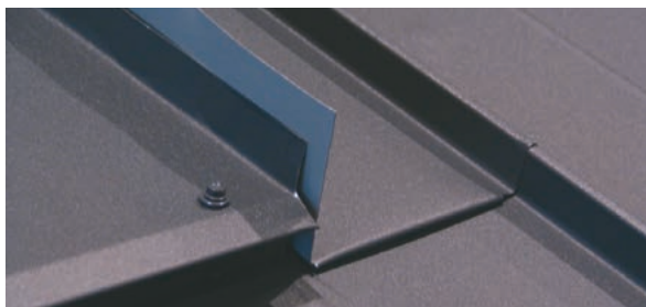
Klempířské spojení čelního oplechování a boční šablony.
