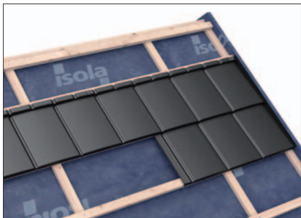
Příklad: pokládka na střih
