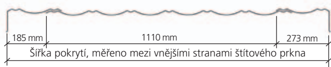
Pokrytá šířka střechy (mm)
