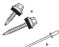
a) Kotvící šrouby SWT a SL2T, b) trhací vodotěsný nýt POP
